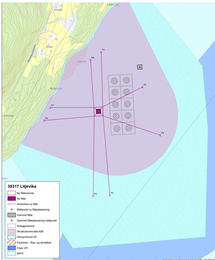
Figur 2: Kartet viser dagens flåteplassering (grå firkant) og omsøkte plassering inkludert ankerlinjer (lilla firkant og linjer). Flåten søkes flyttet sørvest fra anleggets nordøstlige hjørne, og ny plassering vil være mellom anleggsrammen og Dyrøya. Bilde hentet fra søknad.
