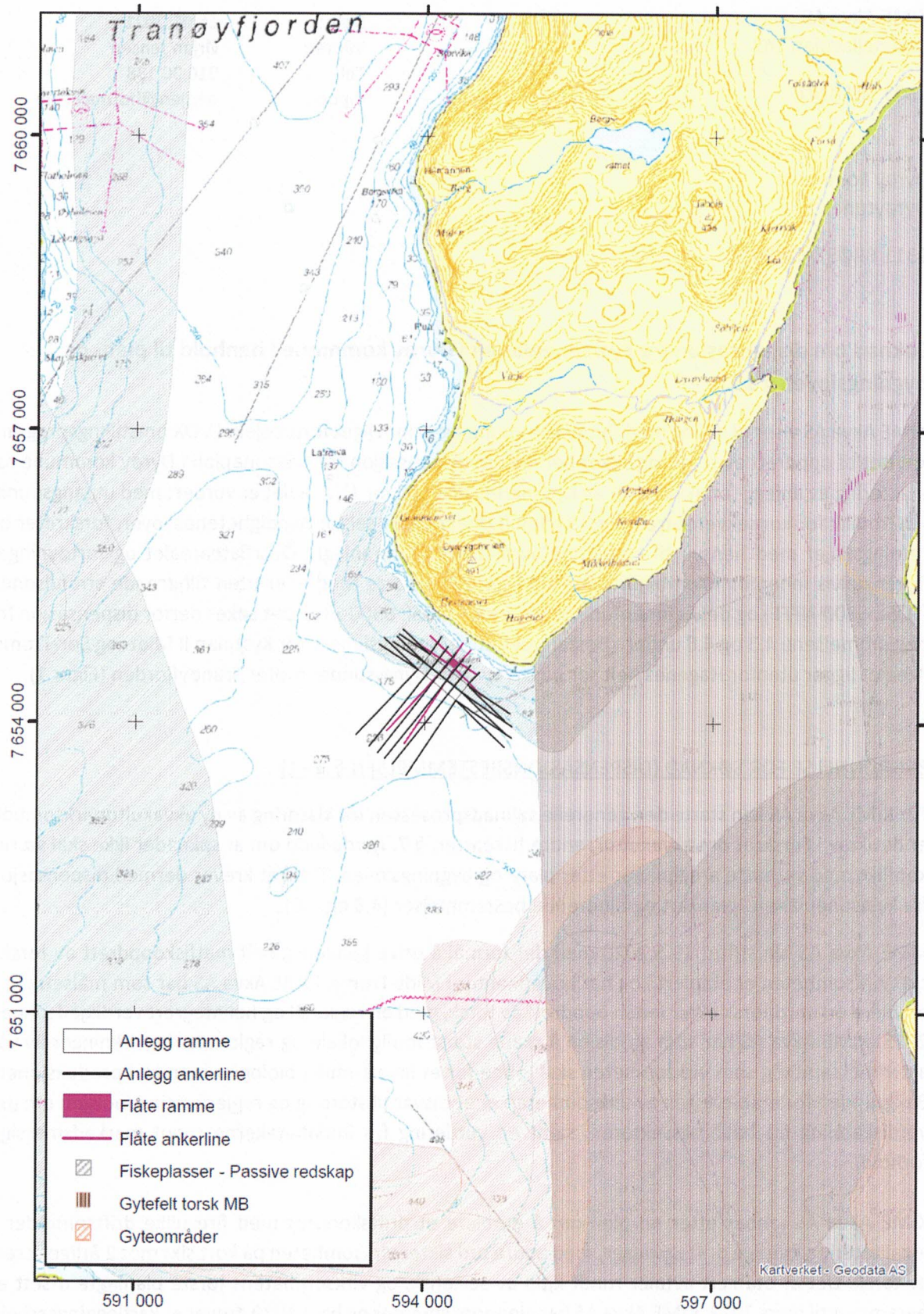
Figur 1: Lokalitet Hagenes, overflateareal og fortøyningslinjer
